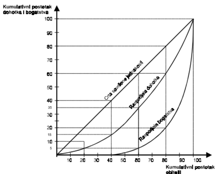
Slika 2. Lorenzova krivulja 40
