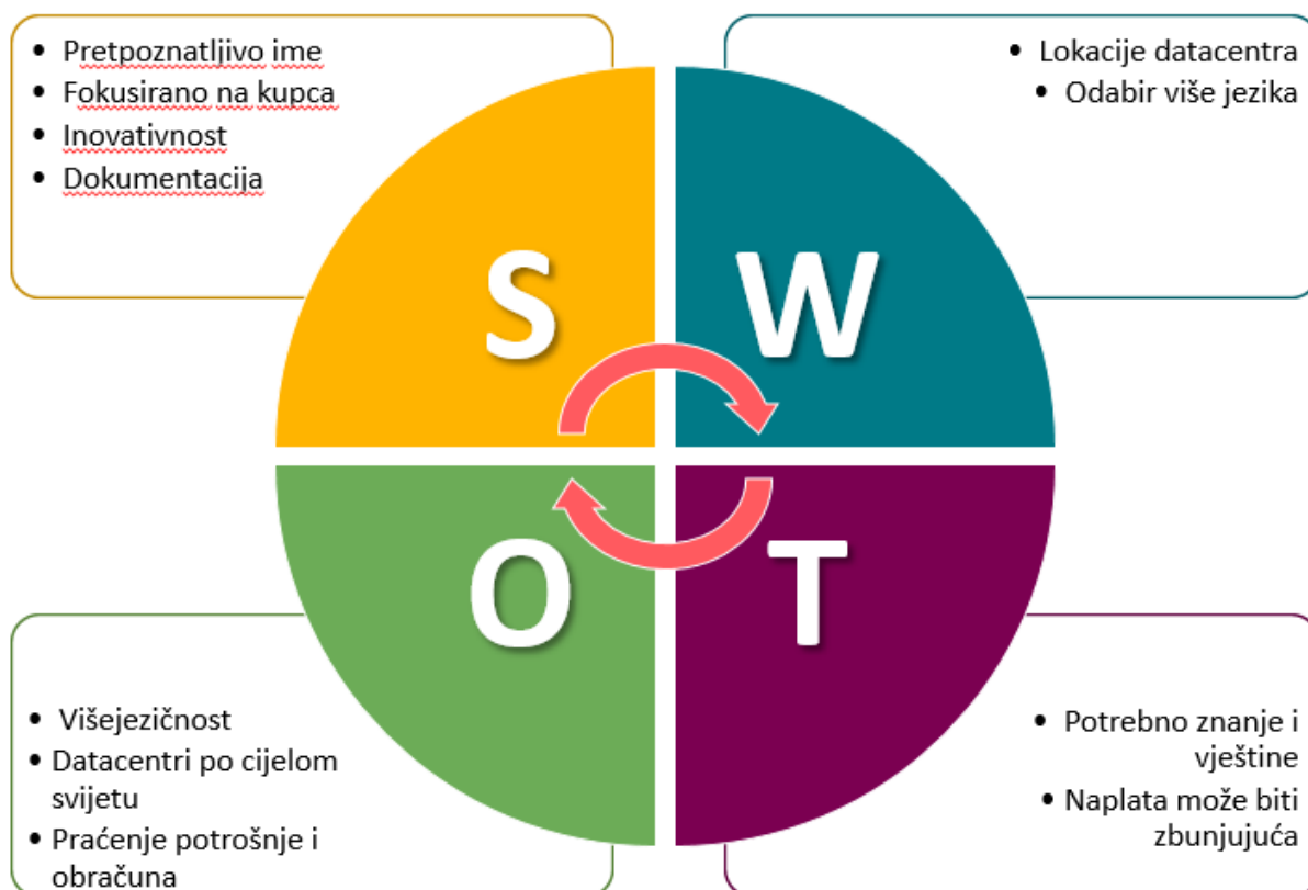
Slika 13: SWOT analiza
