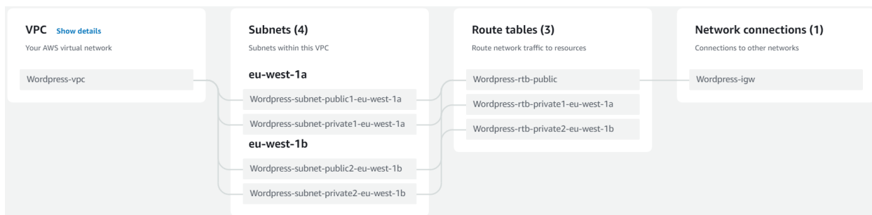
Slika 16: Vizualizacija VPC-a
