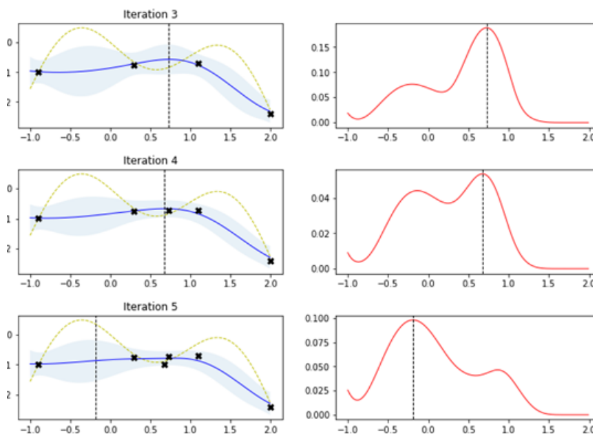
Slika 16: 3., 4. i 5. iteracija Bayesove optimizacije
