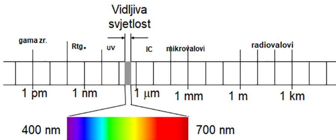
Slika 1. Razlaganje svjetlosti
