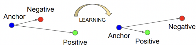
Slika 9.: Trostruki gubitak
