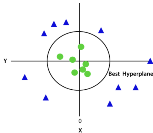
Slika 5.: Nelinearni SVM
