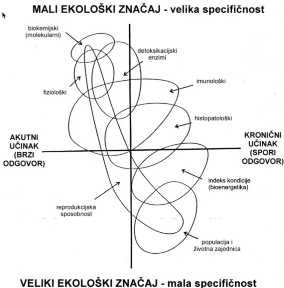
Slika 1. Razine biološkog odgovora organizma na izloženost stresu i zagađivalima u okolišu u ovisnosti o vremenu nastanka učinka i ekološkoj značajnosti (specifičnosti) (Prema Adams i sur., 1989).
