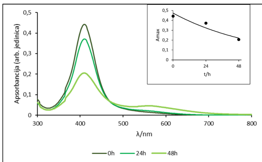
Slika 15. Promjena apsorpcijskog spektra i apsorpcijskog maksimuma humične kiseline ( 1 \mu\text{g/mL} ) i AgNP-a ( 0.02 \mu\text{g/mL} ) snimanog u ultračistoj vodi kroz 48 h.
