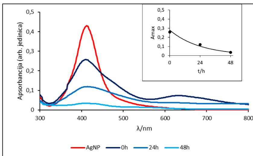
Slika 16. Promjena apsorpcijskog spektra i apsorpcijskog maksimuma humične kiseline ( 1 \mu\text{g/mL} ) i AgNP-a ( 0.02 \mu\text{g/mL} ) snimanog u ASW kroz 48 h.
