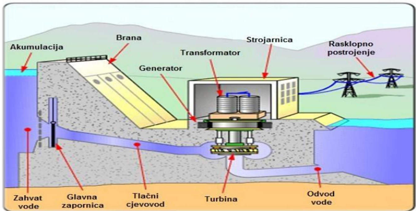
Slika 14. Dijelovi hidroelektrane [11]
