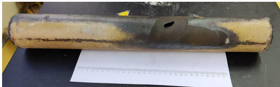
Slika 14: Cijev s pukotinom iz TE Plomin
