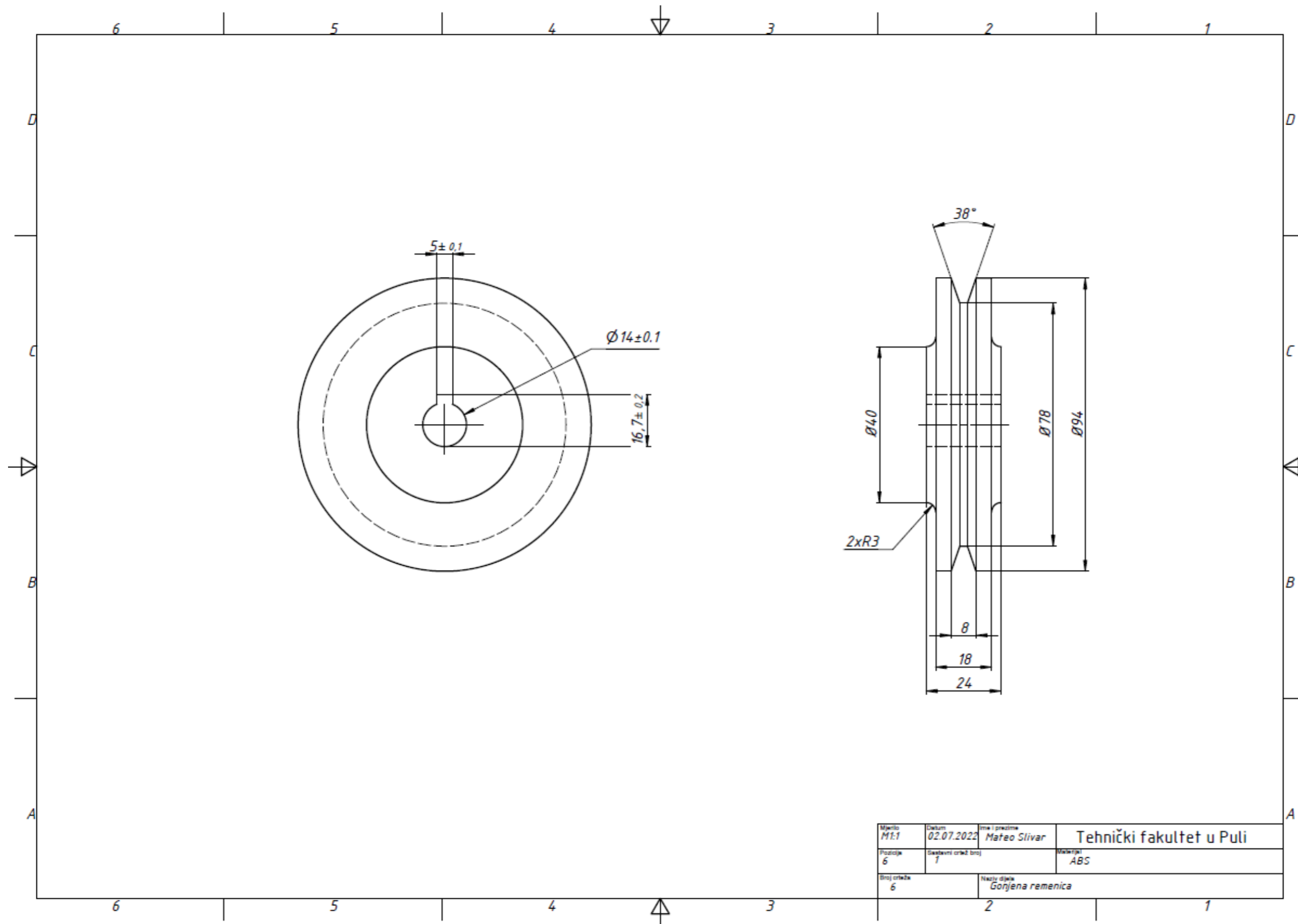
Prilog 1. Radionički crtež gonjene remenice
