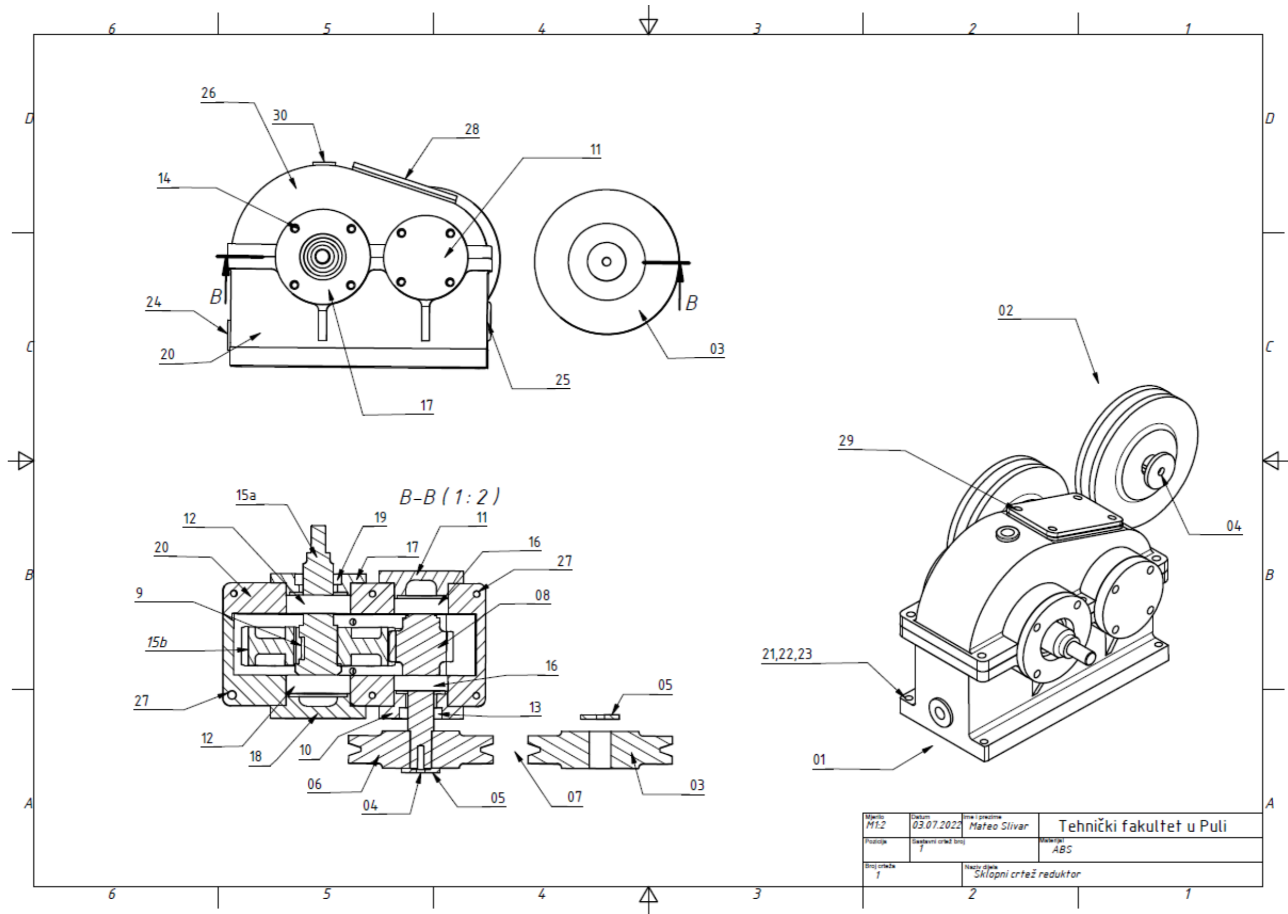
Prilog 11. Sklopni (montažni) crtež reduktora
