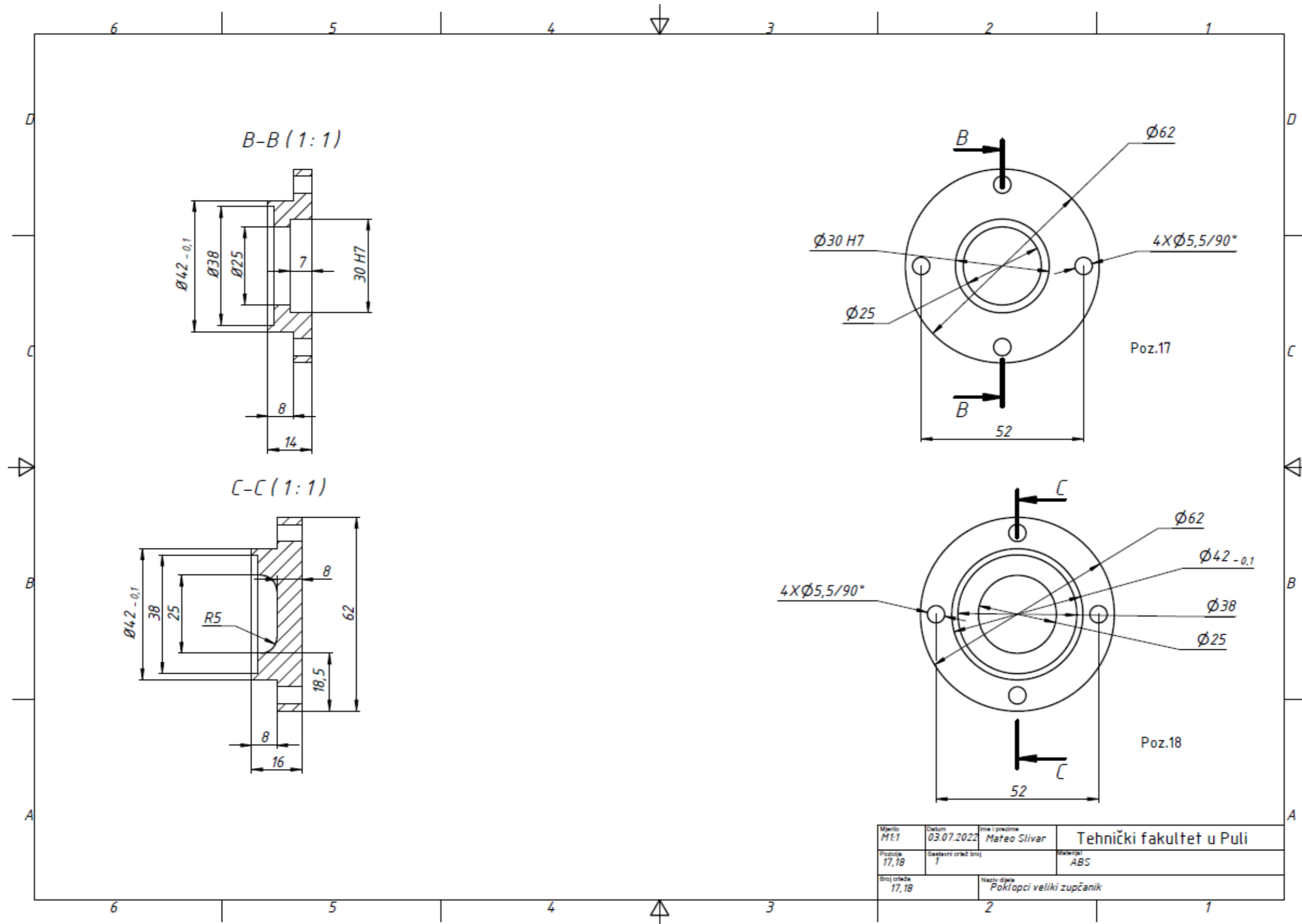
Prilog 4. Radionički crtež poklopaca gonjenog zupčanika
