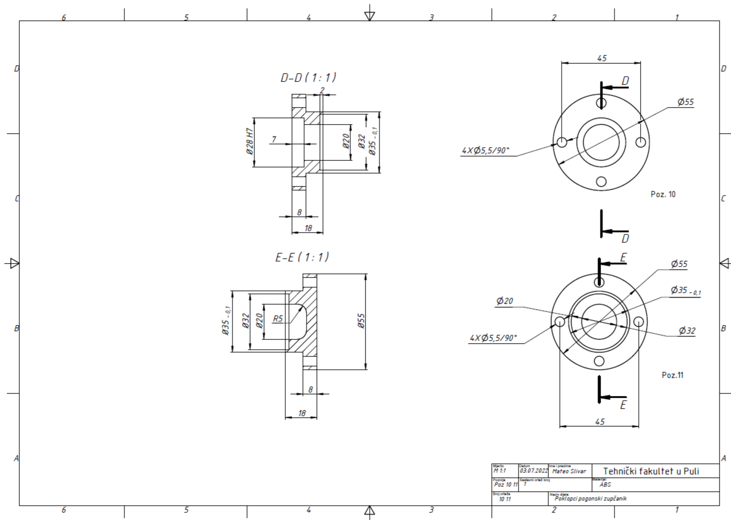
Prilog 3. Radionički crtež poklopca pogonskog zupčanika
