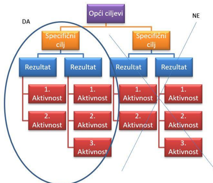
Slika 4. Stablo ciljeva
