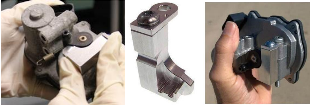
Slika 56: Primjer izvedbe kupovnih nosača specijaliziranih za otklon greške P2015 i mjesto postavljanja
