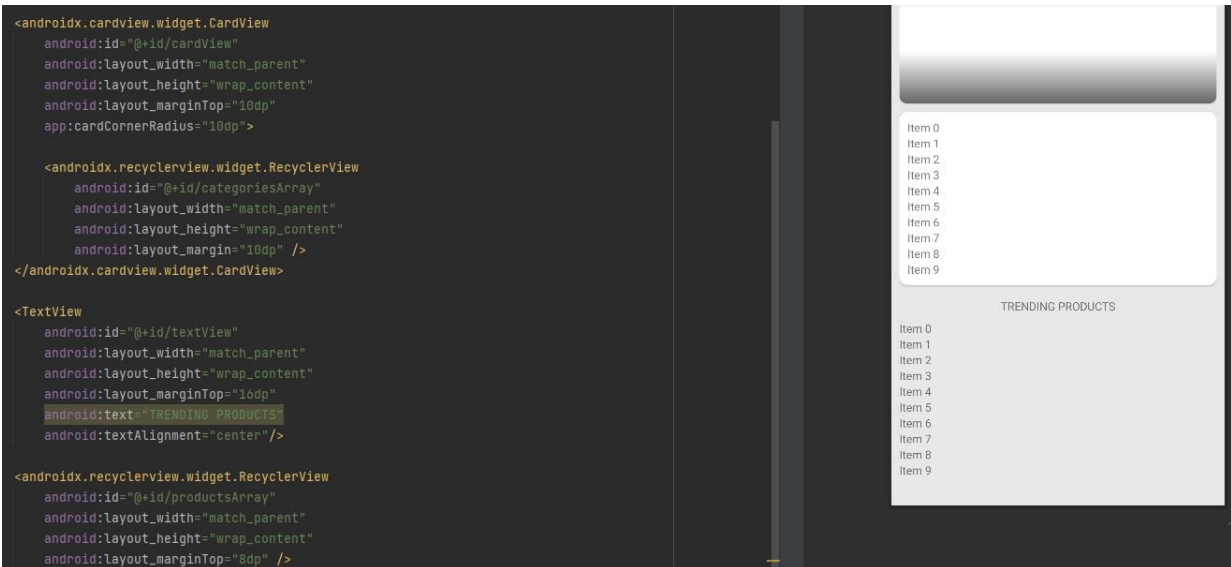
Slika 27. RecyclerView-ovi za kategorije i proizvode u datoteci activity_main.xml
