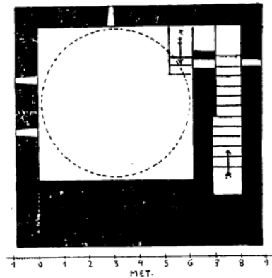
SI 37. Horizontalni presjek prvog kata barutane Mazalić, 1952. str. 77
