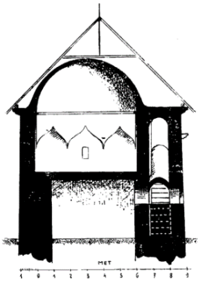
SI 36. Vertikalni presjek barutane Mazalić, 1952. str. 76
