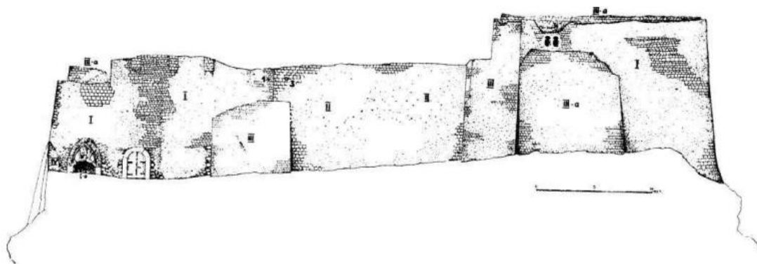
SI 22. Shematski prikaz južnog zida citadele prije konzervacije sa arhitektonskim fazama raspodijeljenih po Basleru Basler, 1959. str. 123
