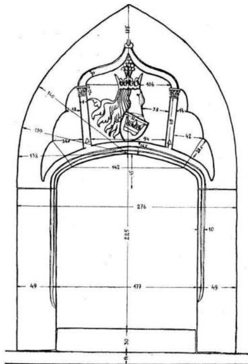
SI 25. Baslerova skica portala sa grbom Basler 1959. str. 126
