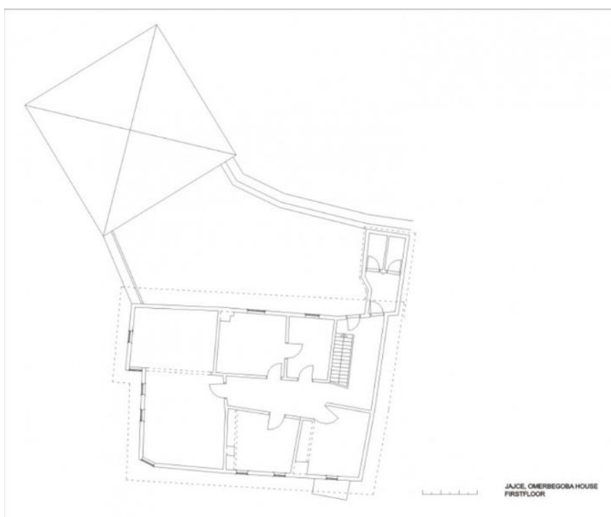
SI 51. Prikaz tlocrta bastiona s Travničkom kapijom i Omer-begovom kućom
