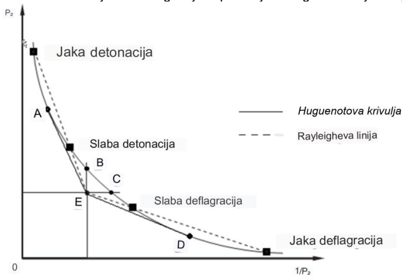
Slika 25. Detonacijsko i deflagacijsko područje u Huguenotovoj krivulji.
