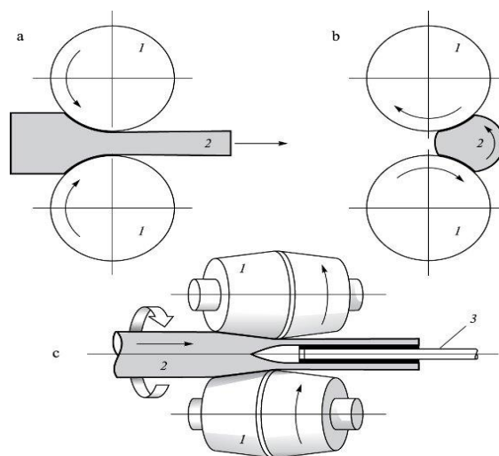
Slika 5: Vrste valjanja
