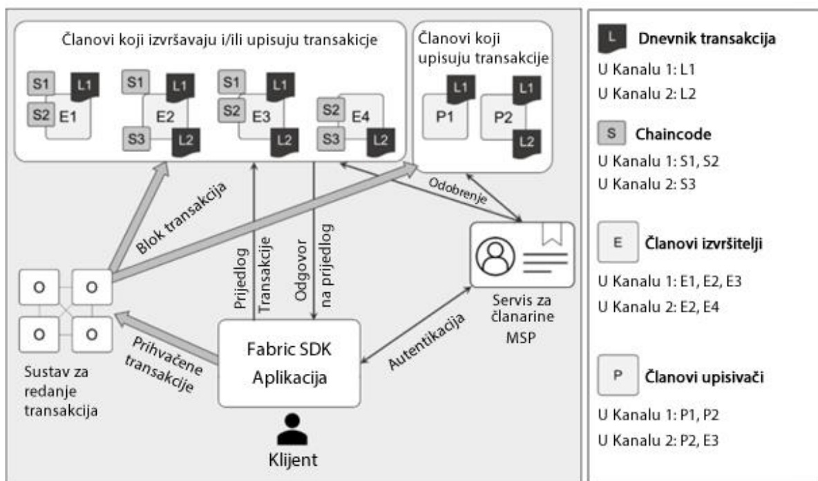
Slika 9. Prikaz transakcijskog procesa unutar Hyperledger Fabric mreže.
