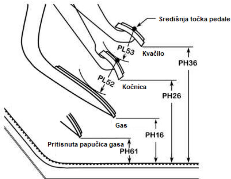
Slika 16: Visina pedala i udaljenost od poda
