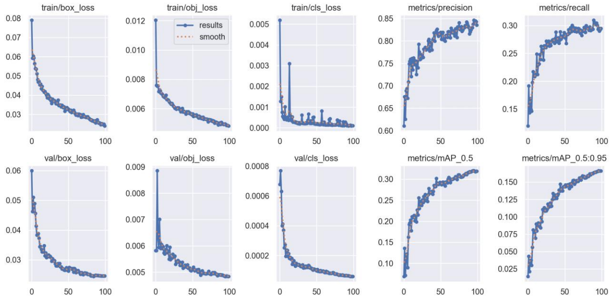
Slika 33 - Prikaz kretanja vrijednosti svih metrika po epochama kroz proces treniranja More50 modela
