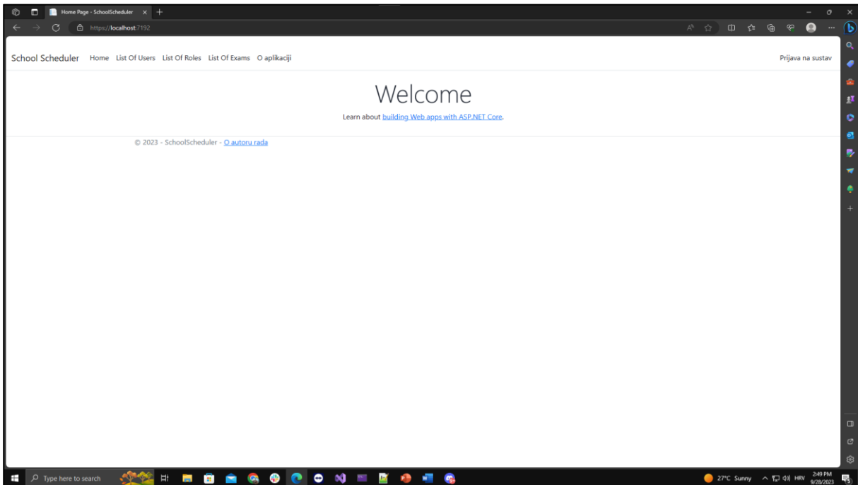
Slika 5 Pregled ekrana
