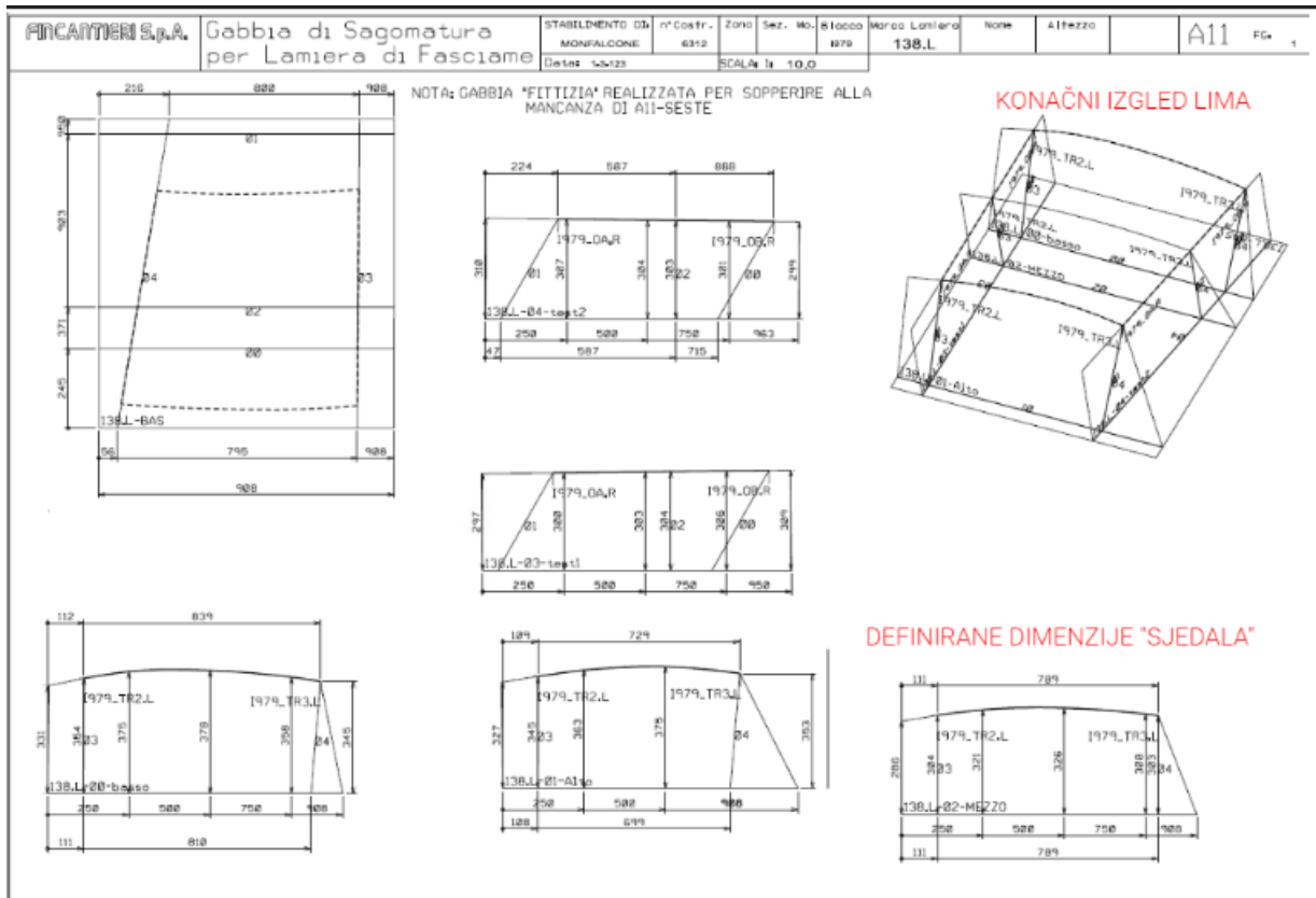
Slika 31: Tehnička dokumentacija savijanja limova
