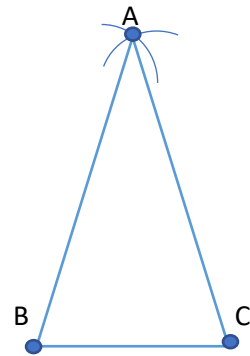
Slika 11. Jednakokračni trokut
