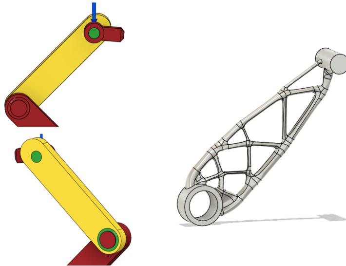
Slika 45 Generativni dizajn robotske ruke 4/4
