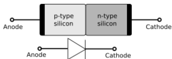
Slika 21. P-n spoj
