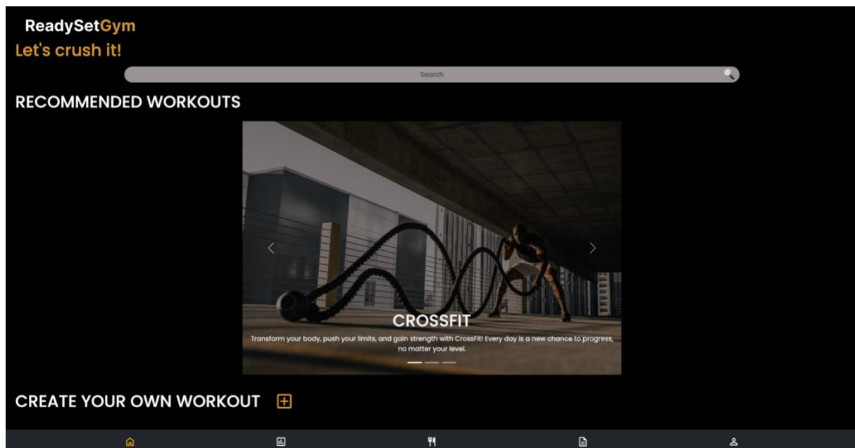
Slika 9. Prikaz homepage-a
