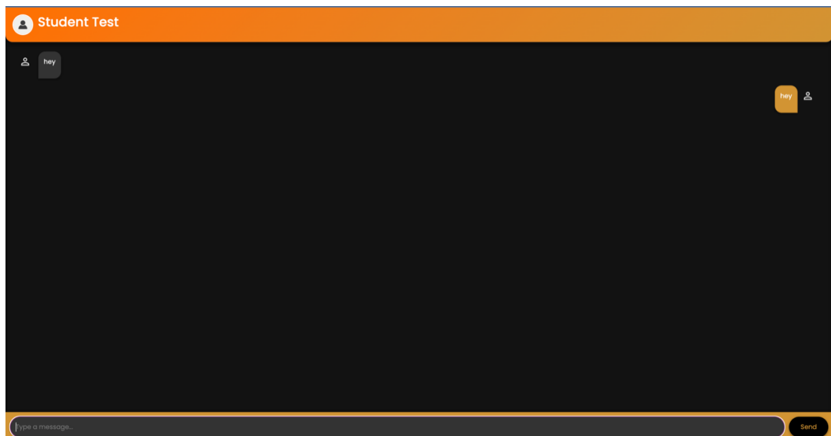
Slika 18. Prikaz chat-a
