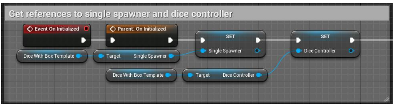
Slika 38. Dohvaćanje referenci iz DiceWithBoxTemplate instance preko funkcije OnInitialized() unutar klase DiceTemplate.
