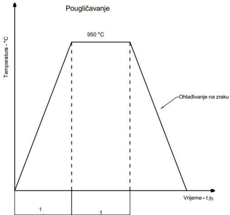
Slika 7.5. - Proces pouglčavanja strojnog dijela svornjak
