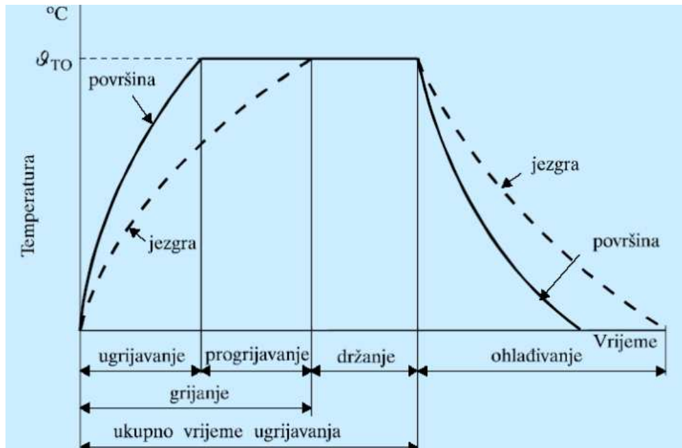
Slika 2.1 – dijagram odnosa vremena i temperature
