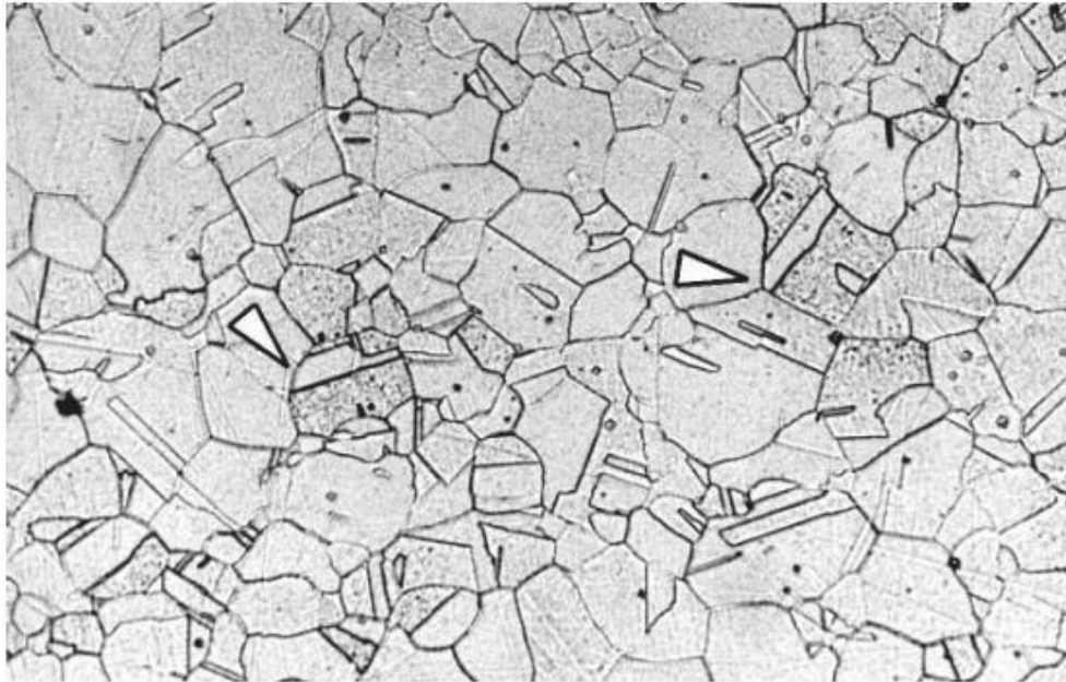
Slika 3.1. – mikrostruktura austenita
