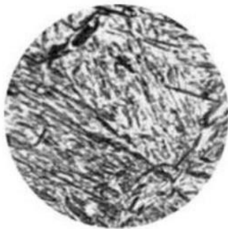
Slika 3.5. - Mikrostruktura martenzita
