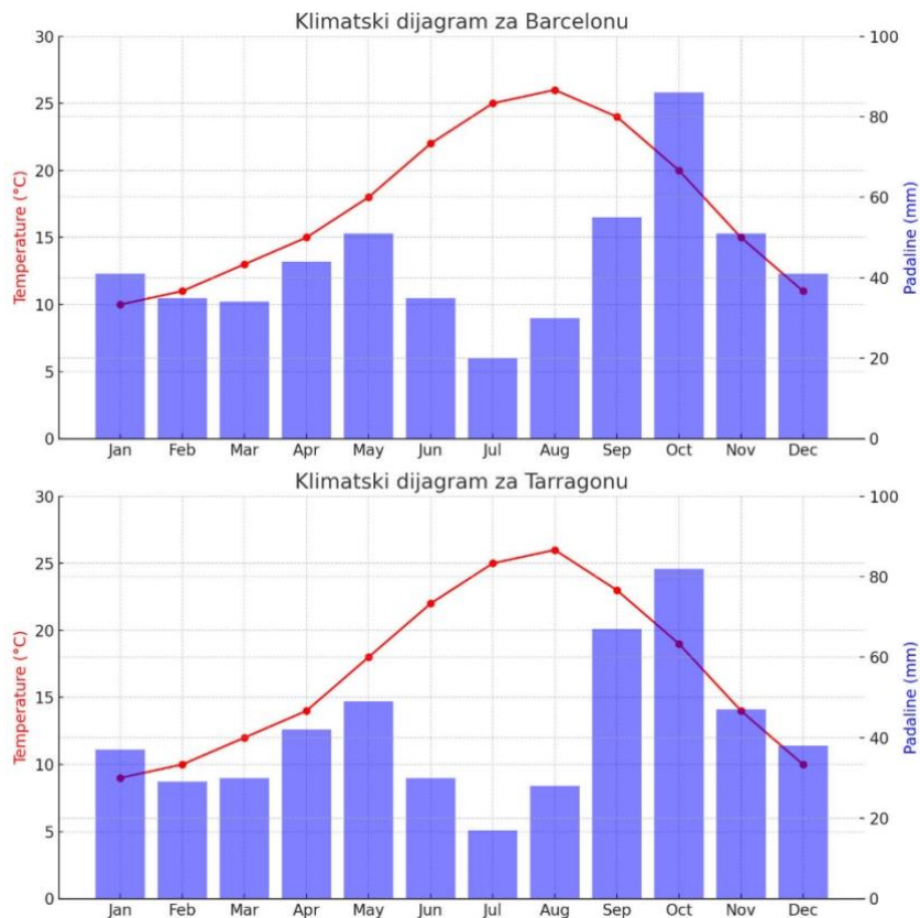
Slika 2. Prikaz klimatskog dijagrama Barcelone i Tarragone
